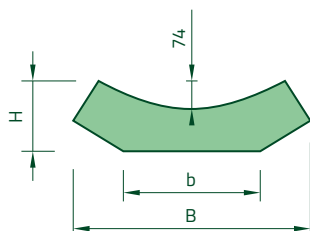
odvodňovací žlab C
