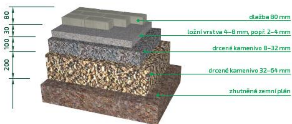
Obr 2. Příklad skladby jezdové plochy pro vozidla do 3,5 t
