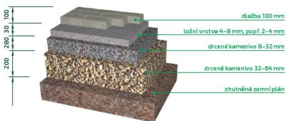
Obr 3. Příklad skladby jezdové plochy pro vozidla nad 3,5 t
