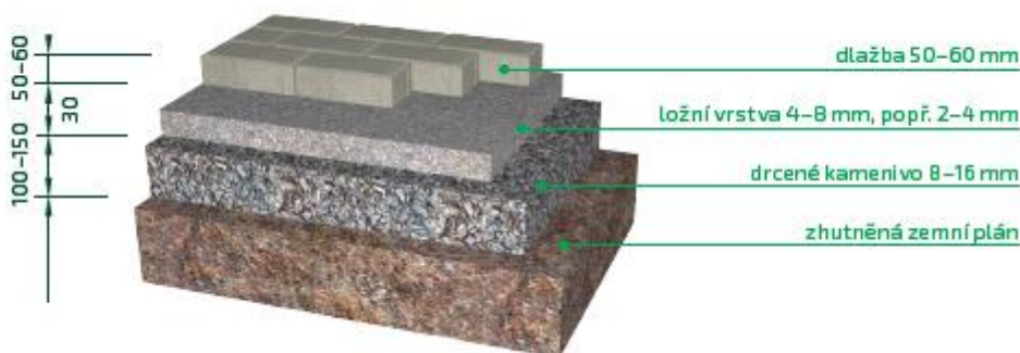
Obr 1. Příklad skladby chodníku
